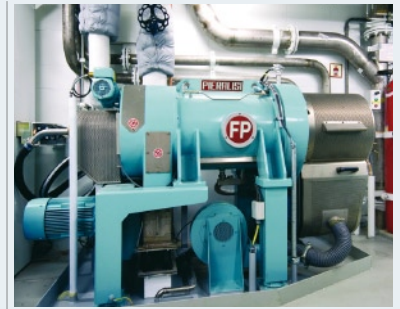
Trattamento fanghi biologici su navi da crociera - Biological sludge treatment on cruise ship - Elimination des boues biologiques sur bateau de croisière
